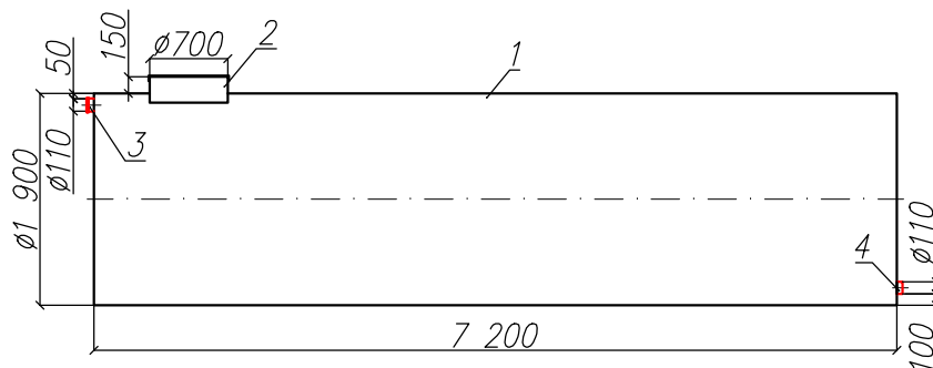
Разрез 1-1
