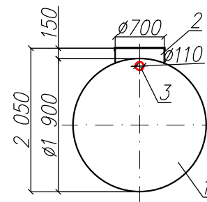
Вид спереди
